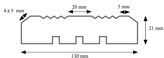
1 face striée avec un plat de 20 mm au milieu et 1 plat de 5 mm de chaque côté. 2 chanfreins de 4 à 5 mm | 3 rainures de détente
