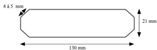
2 faces lisses | 4 chanfreins de 4 à 5 mm
