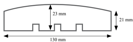
1 face bombée | 3 rainures de détente
