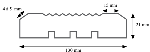
1 face striée avec un plat de chaque côté de 15 mm 2 chanfreins de 4 à 5 mm | 3 rainures de détente
